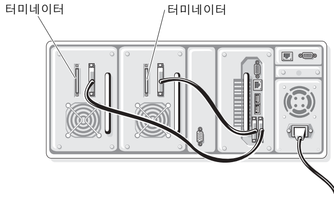
그림 1-19. 2 개 드라이브로 구성된 테이프 라이브러리
